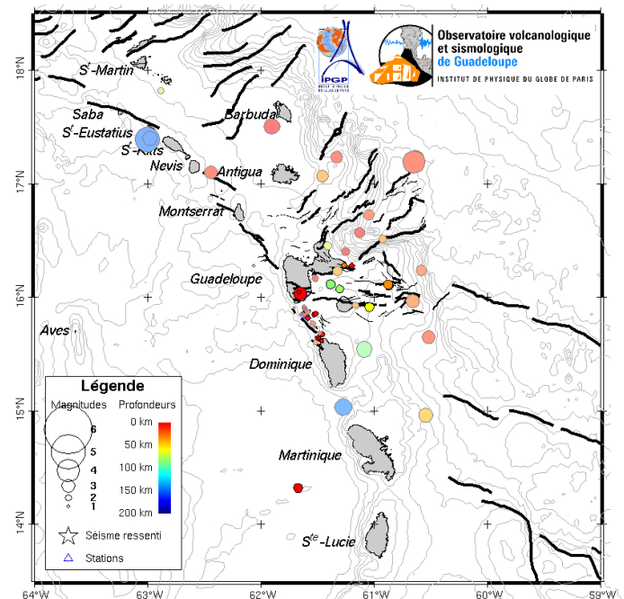
Figure 1. Carte des épïcêtres du mois de mars 2013 correspondant aux séismes enregistrés et localisés par l'OVSG-IPGP dans un rayon de 450 km autour de la Guadeloupe. Traits noirs = failles principales connues (d'après Feuillet et al. 2000).
