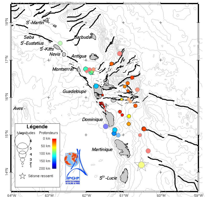
Figure 1. Carte des épacentres du mois de décembre 2012 correspondant aux séismes enregistrés et localisés par l'OVSG-IPGP dans un rayon de 450 km autour de la Guadeloupe. Traits noirs = failles principales connues (d'après Feuillet et al. 2000).
