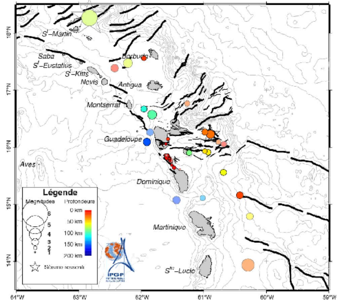
Figure 1. Carte des épacentres du mois de juillet 2012 correspondant aux séismes enregistrés et localisés par l'OVSG-IPGP dans un rayon de 450 km autour de la Guadeloupe. Traits noirs = failles principales connues (d'après Feuillet et al. 2000).
