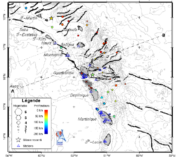
Figure 1. Carte des épacentres du mois de mars 2010 correspondants aux séismes enregistrés et localisés par l'OVSG-IPGP dans un rayon de 450 km autour de la Guadeloupe (voir la légende). Traits noirs = failles principales connues (d'après Feuillet et al. 2000).
