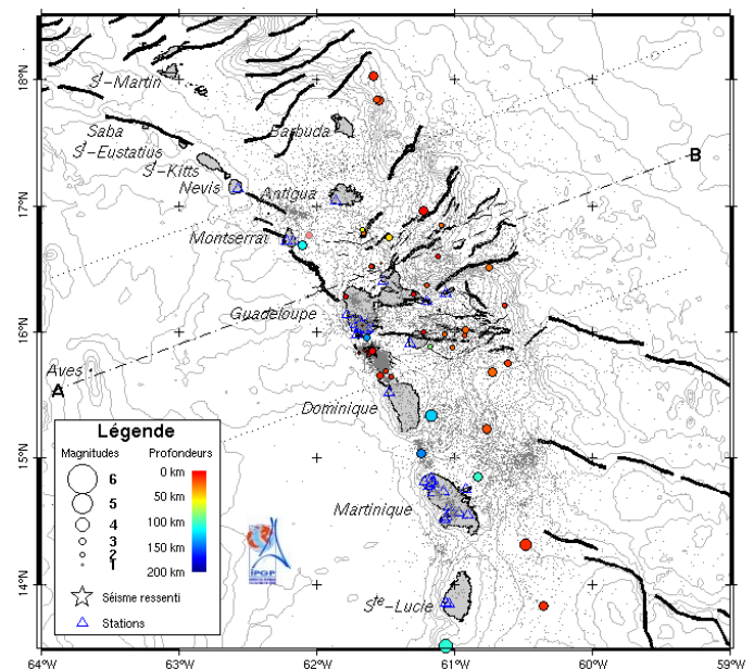
Figure 1. Carte des épacentres du mois de septembre 2009 correspondants aux séismes enregistrés et localisés par l'OVSG-IPGP (voir la légende). Traits noirs = failles principales connues (d'après Feuillet et al. 2000).
