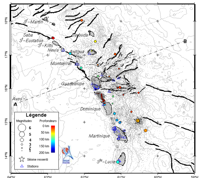
Figure 1. Carte des épacentres du mois d'août 2009 correspondant aux séismes enregistrés et localisés par l'OVSG-IPGP (voir la légende). Traits noirs = failles principales connues (d'après Feuillet et al. 2000).
