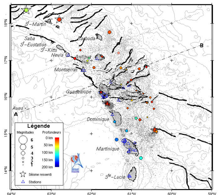
Figure 1. Carte des épacentres du mois de mai 2009 correspondants aux séismes enregistrés et localisés par l'OVSG-IPGP (voir la légende). Traits noirs = failles principales connues (d'après Feuillet et al. 2000).
