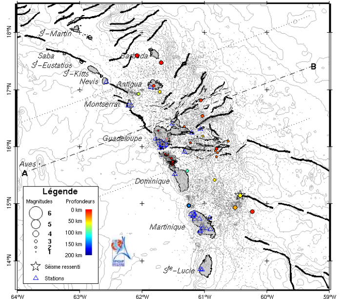
Figure 1. Carte des épïcêtres du mois d'avril 2009 correspondants aux séismes enregistrés et localisés par l'OVSG-IPGP (voir la légende). Traits noirs = failles principales connues (d'après Feuillet et al. 2000).
