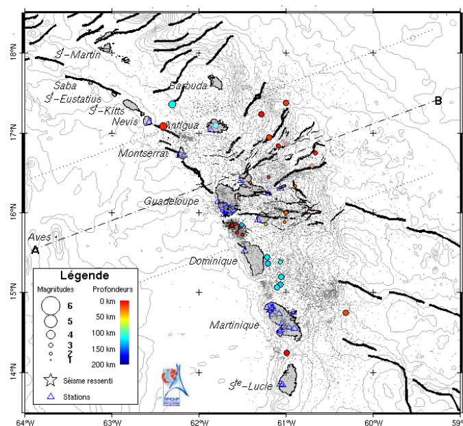
Figure 1. Carte des épicentres du mois de janvier 2009 correspondant aux séismes enregistrés et localisés par l'OVSG-IPGP (voir la légende). Traits noirs = failles principales connues (d'après Feuillet et al. 2000).
