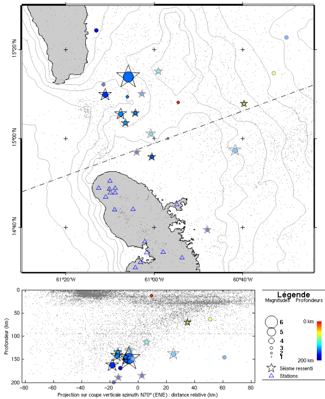
Figure 3. Carte des épencentres du mois de décembre 2007 correspondants aux séismes enregistrés et localisés par l'OVSG-IPGP en Martinique (voir la légende). Traits gris = courbes bathymétriques.
