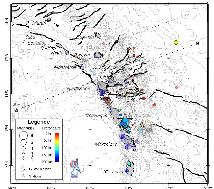
Figure 1. Carte des épicentres du mois de décembre 2007 correspondants aux séismes enregistrés et localisés par l'OVSG-IPGP (voir la légende). Traits noirs = failles principales connues (d'après Feuillet, 2000), traits gris = courbes bathymétriques.
