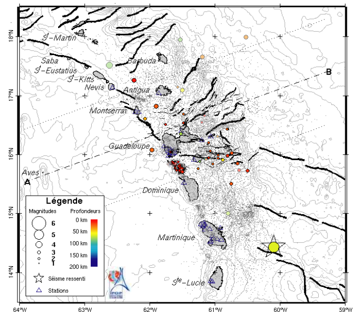
Figure 1. Carte des épacentres du mois de septembre 2007 correspondant aux séismes enregistrés et localisés par l'OVSG-IPGP (voir la légende). Traits noirs = failles principales connues (d'après Feuillet, 2000), traits gris = courbes bathymétriques.
