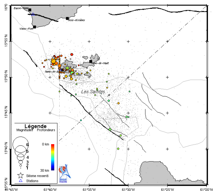
Figure 3. Localisations préliminaires des 107 principales répliques du mois de décembre 2006 : traits noirs = failles connues, traits gris = courbes bathymétriques, petits points gris = épicentres de tous les séismes connus.
