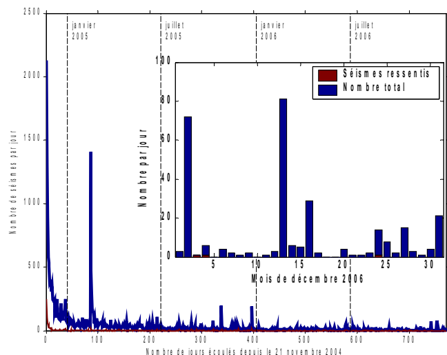
Figure 2. Évolution du nombre de séismes (répliques des Saintes) entre le 21 novembre 2004 et le 31 décembre 2006 (771 ème jour de répliques) : estimations du nombre de séismes potentiellement ressentis et nombre total par jour. Encart : détail des données sur le mois de décembre 2006.
