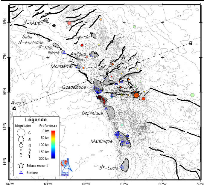
Figure 1. Carte des épicentres du mois de décembre 2006 correspondant aux séismes enregistrés et localisés par l'OVSG-IPGP. Traits noirs = failles principales connues, traits gris = courbes bathymétriques.
