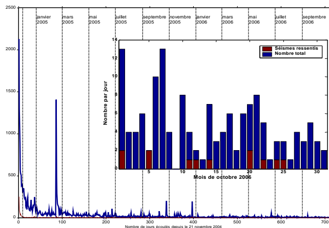
Figure 2. Évolution du nombre de séismes (répliques des Saintes) entre le 21 novembre 2004 et le 31 octobre 2006 (710 ème jour de répliques) : estimations du nombre de séismes potentiellement ressentis et nombre total par jour. Encart : détail des données sur le mois d'octobre 2006.
