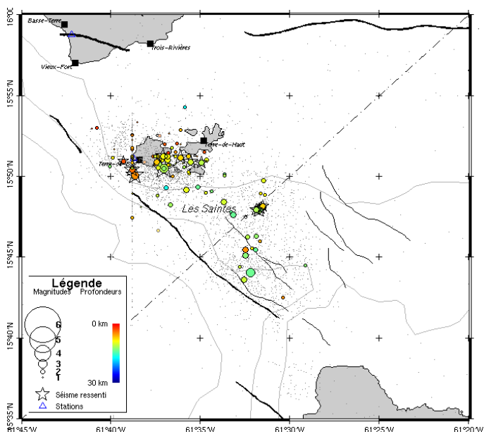
Figure 3. Localisations préliminaires des 123 principales répliques des mois d'octobre 2006 : traits noirs = failles connues, traits gris = courbes bathymétriques, petits points gris = épencentres de tous les séismes connus.
