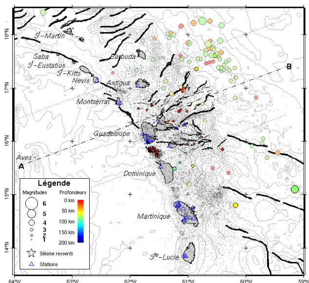
Figure 1. Carte des épïcêtres du mois de octobre 2006 correspondant aux séismes enregistrés et localisés par l'OVSG-IPGP. Traits noirs = failles principales connues, traits gris = courbes bathymétriques.
