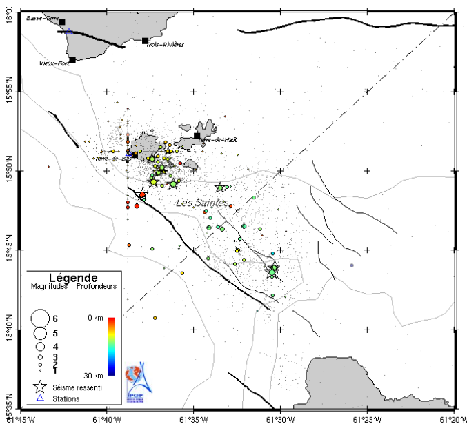
Figure 3. Localisations préliminaires des 192 principales répliques du mois de mai 2006 : traits noirs = failles connues, traits gris = courbes bathymétriques, petits points gris = epicentres de tous les séismes connus.
