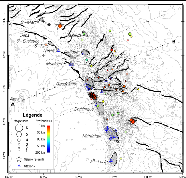
Figure 1. Carte des épicentres du mois de mai 2006 correspondant aux séismes enregistrés et localisés par l'OVSG-IPGP. Traits noirs = failles principales connues, traits gris = courbes bathymétriques.
