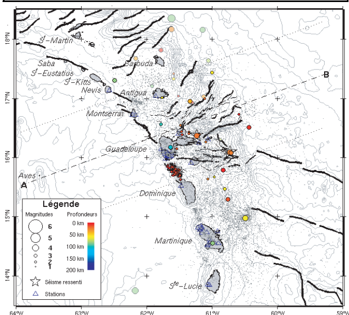
Figure 1. Carte des épicentres du mois de mars 2006 correspondant aux séismes enregistrés et localisés par l'OVSG-IPGP. Traits noirs = failles principales connues, traits gris = courbes bathymétriques.
