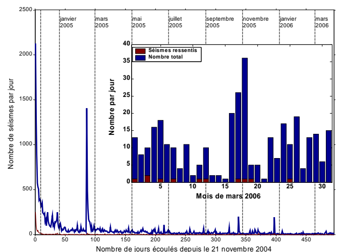
Figure 2. Évolution du nombre de séismes (répliques des Saintes) entre le 21 novembre 2004 et le 31 mars 2006 (495 ème jour de répliques) : estimations du nombre de séismes potentiellement ressentis et nombre total par jour. Encart : détail des données sur le mois de mars 2006.
