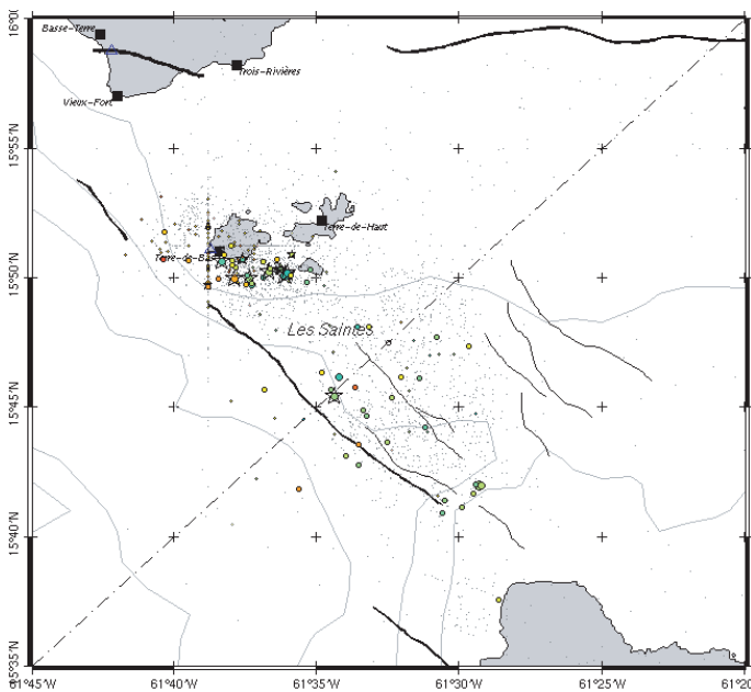
Figure 3. Localisations préliminaires des 199 principales répliques du mois de mars 2006 : traits noirs = failles connues, traits gris = courbes bathymétriques, petits points gris = épacentres de tous les séismes connus.
